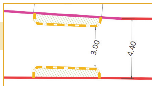
Exemples d'aménagements avec chicane(s)
